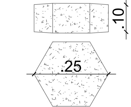
DETALHE BLOCO INTERTRAVADO SEXTAVADO 25X25 SEM ESCALA
