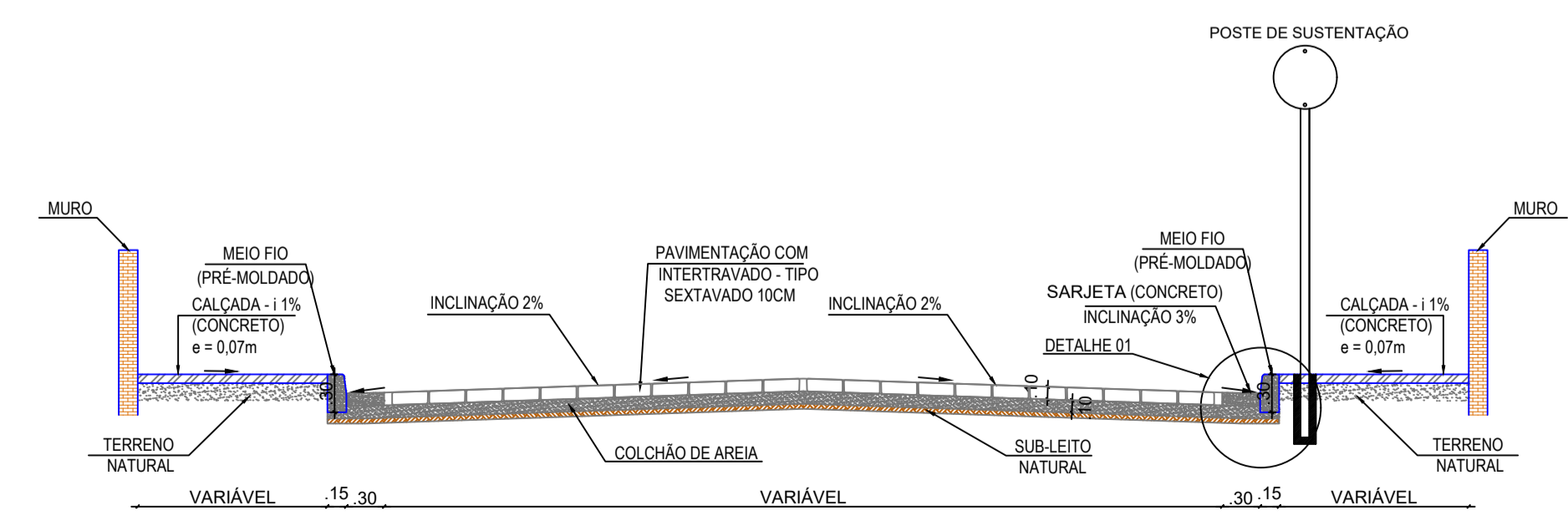
CORTE TRANSVERSAL - Calçada de 1,50 m ESCALA: 1/50
